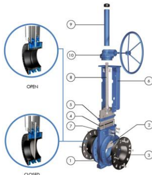
Valve guillotine à boue Slurry knife gate valve
